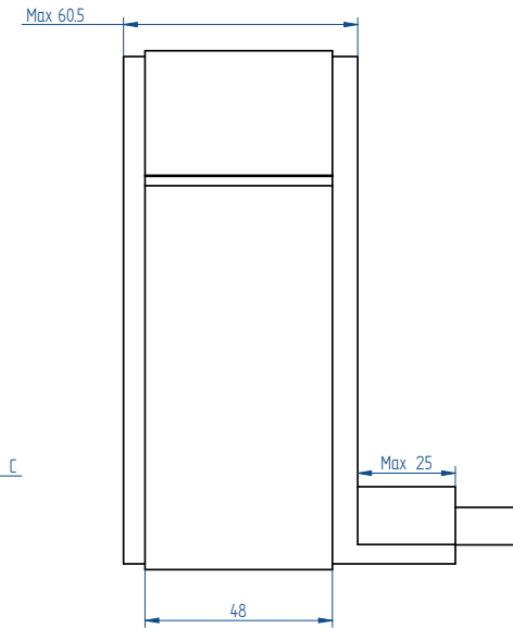
QTR-A 133-60
