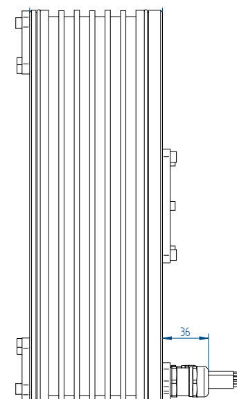
QTL-A 310-105
