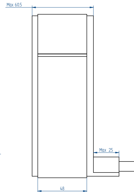
QTR-A 160-60
